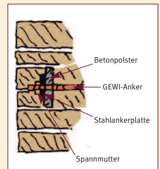
Systemskizze Spannweiterlager.
