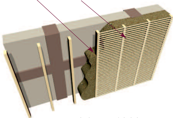
Innenschale aus Leichtlehm
