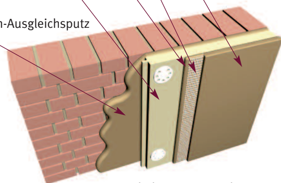
Innenschale aus Dämmplatten
